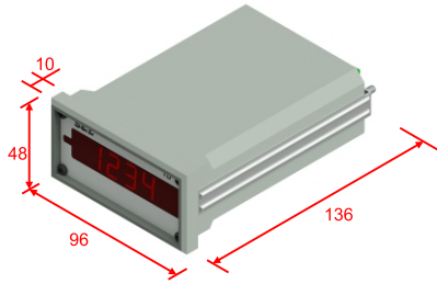
CAIXA 48 x 96 mm
